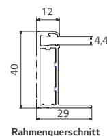
Rahmenquerschnitt
